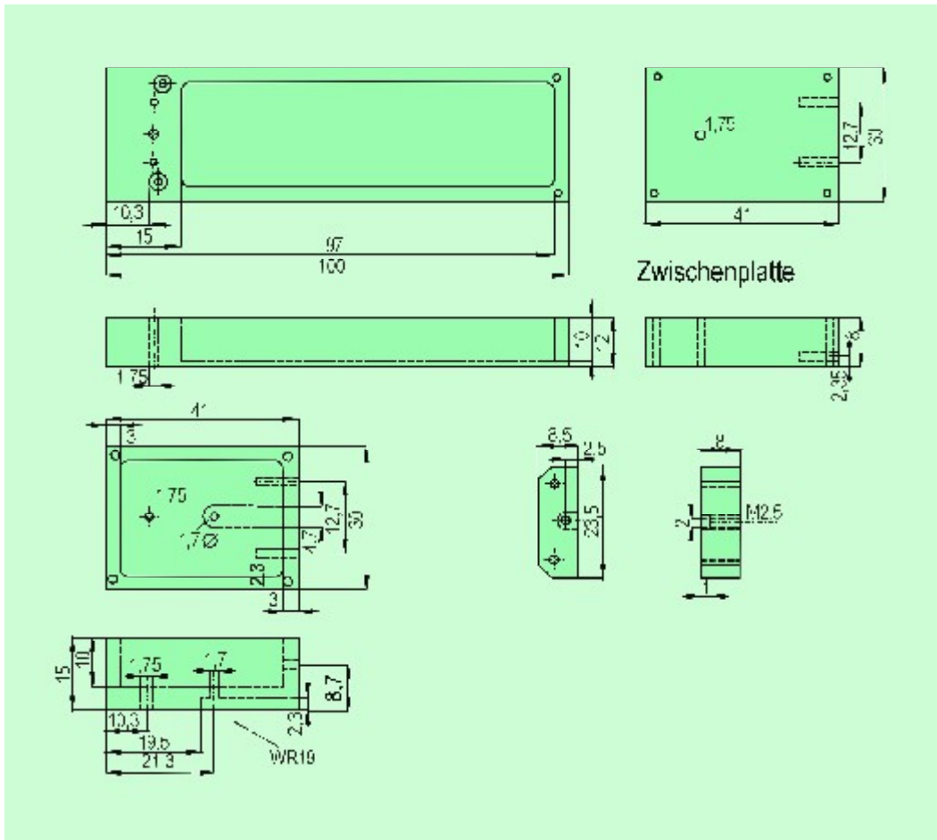
Bild 11: Gehäusezeichnungen
