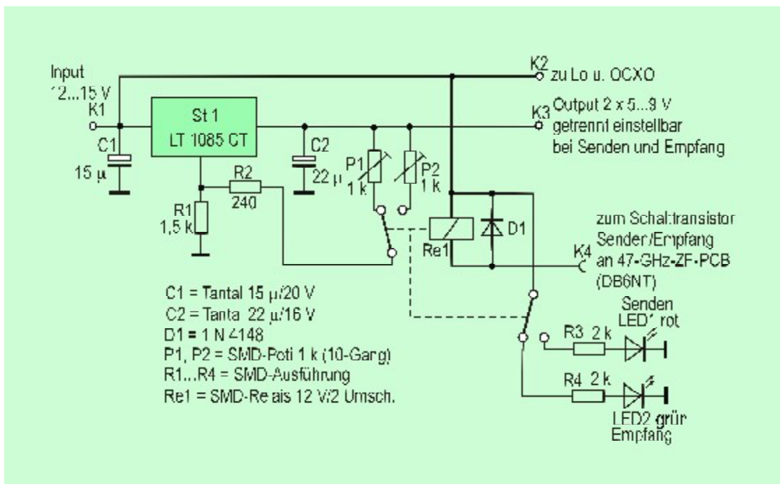
Bild 12: Stromlaufplan
